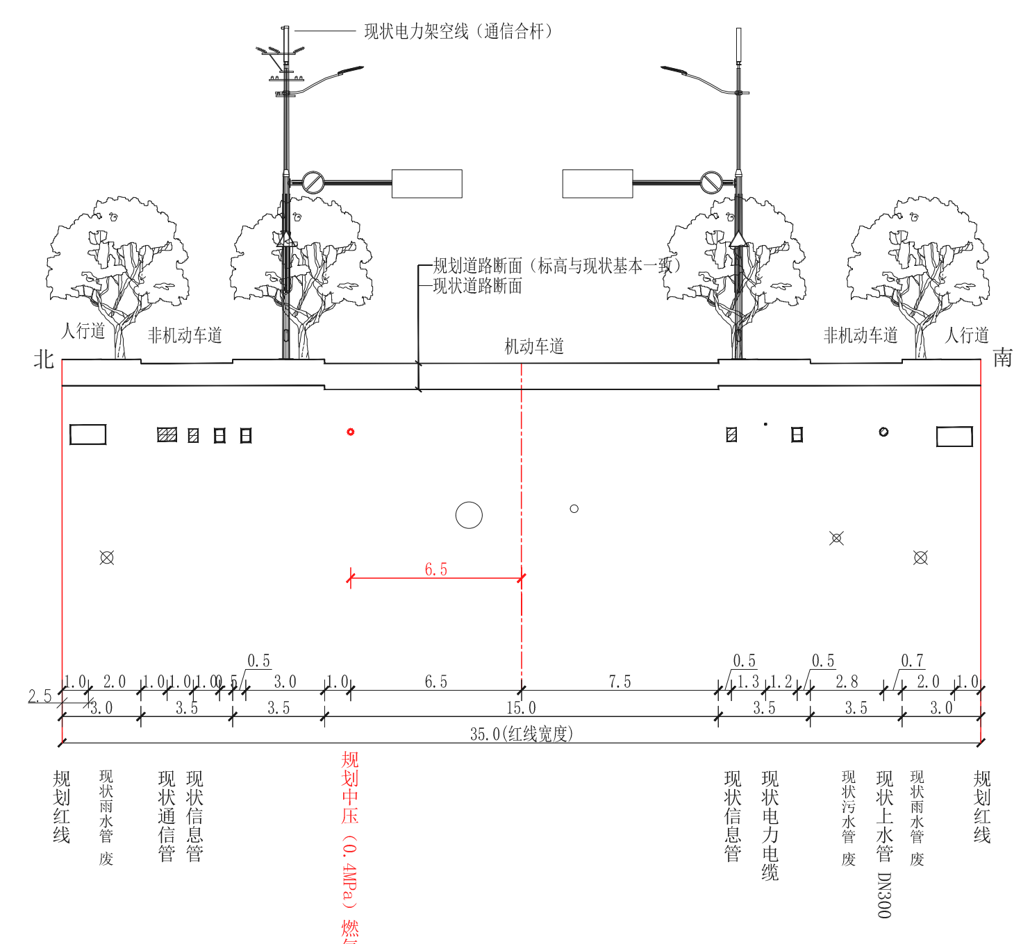
武威路(区界-金迎路)A-A断面图(2023.6.29) 1:200 上海普邑城市规划设计股份有限公司
