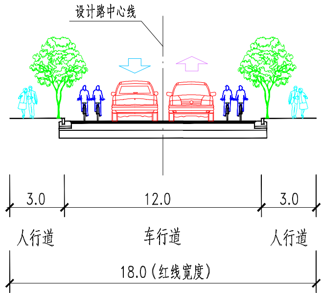
道路标准横断面一 (金昌路~古浪路) 1:200
