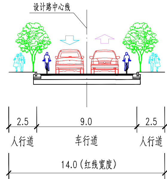
道路标准横断面二 (古浪路~桃惠路) 1:200
