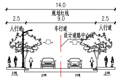
莫高路标准横断面图 1:250
