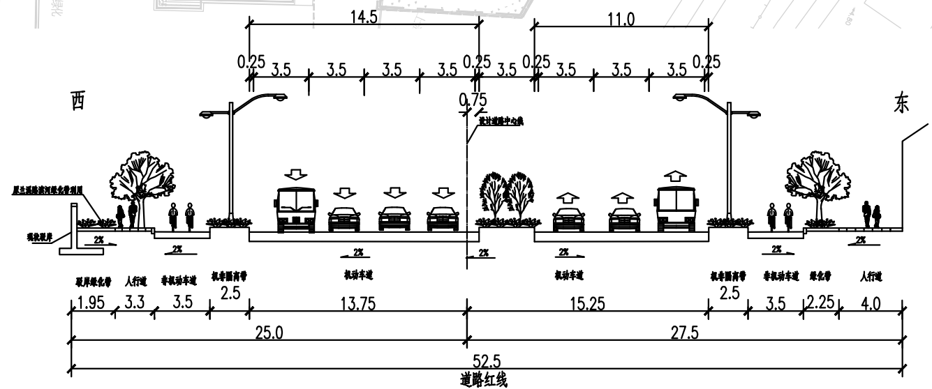
兰溪路(桃浦路以北段)道路横断面图
