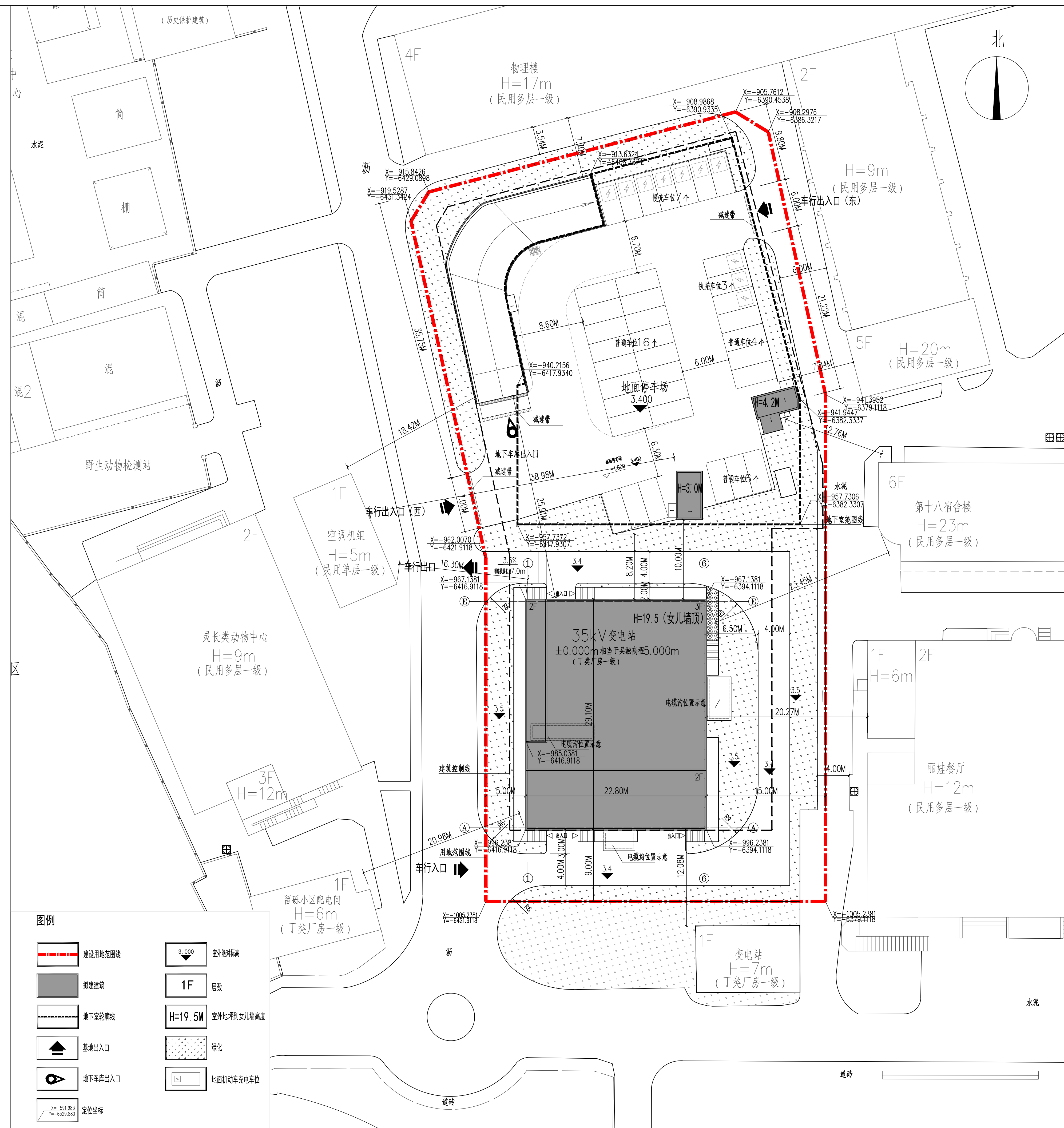
总平面图 1:500
