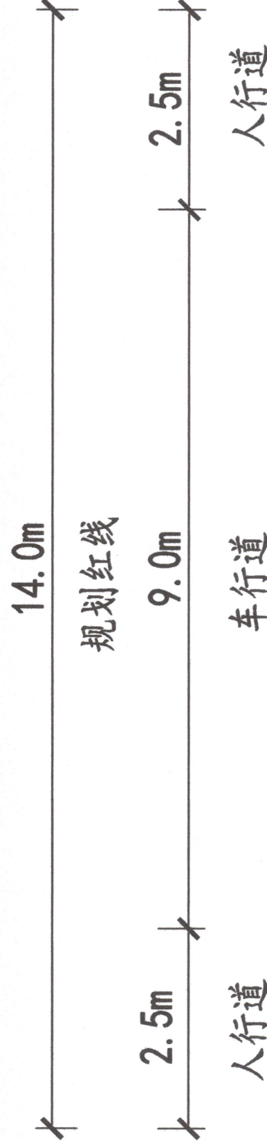
桥梁标准横断面 (2a-2a) 翰景路 (古浪路~武威路)
