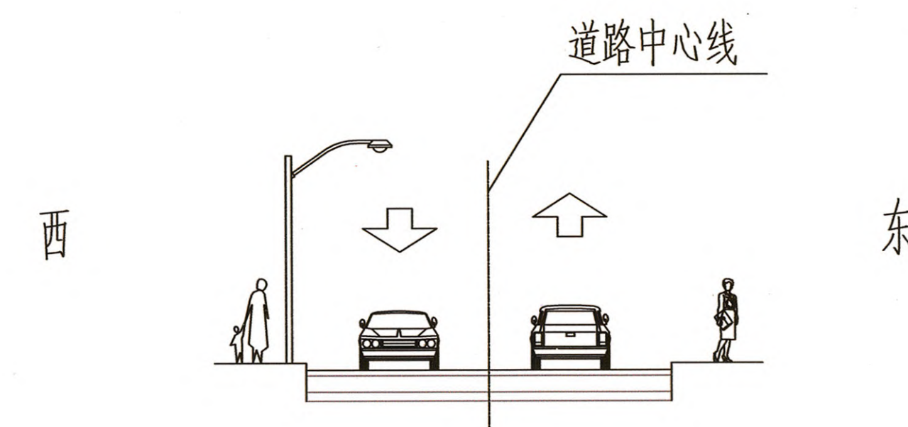
碌曲路(中山北路-堰门路) 道路标准横断面(12m)
