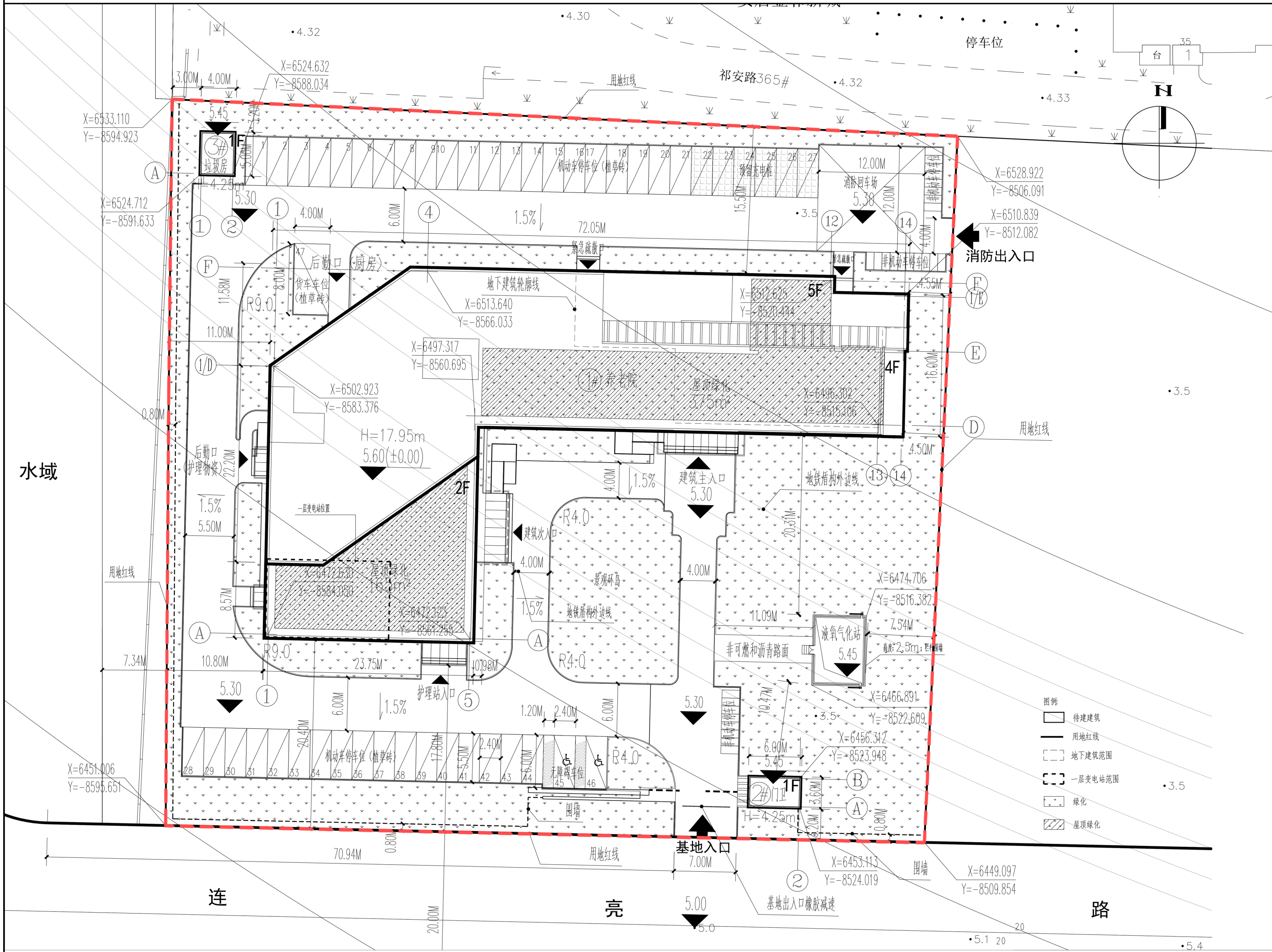
总平面图1:300
