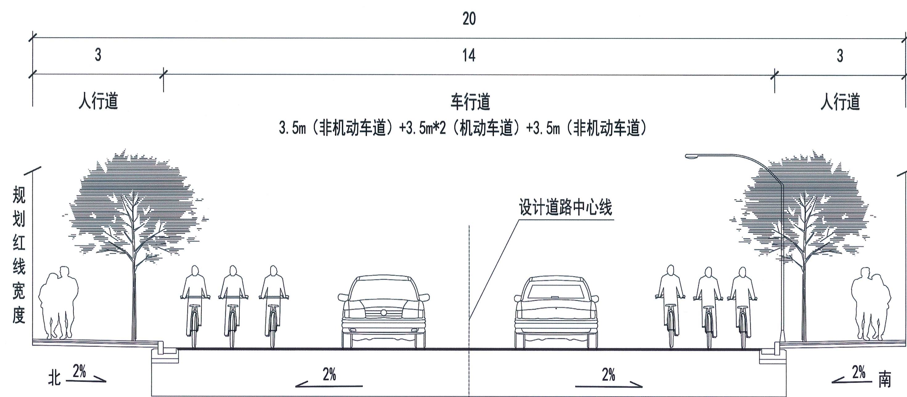
道路标准横断面设计图
