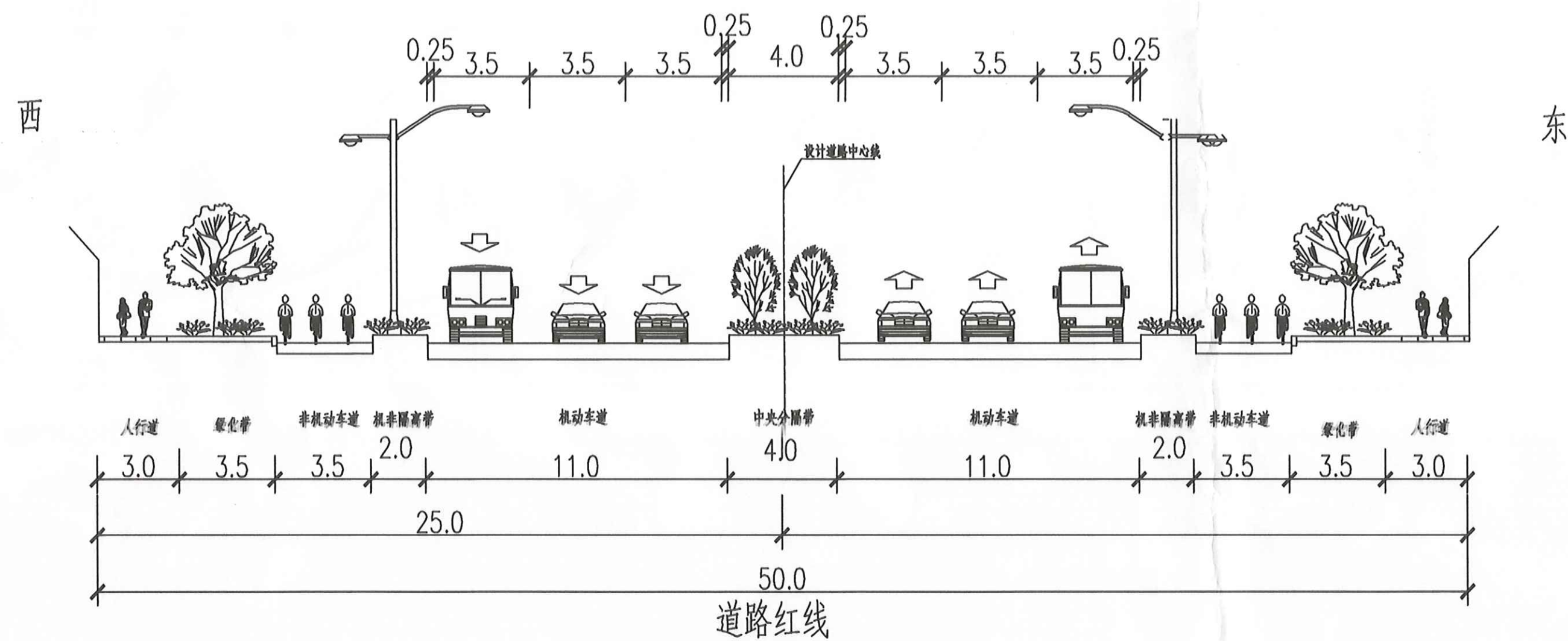
真南路(富平路至新村路)地面道路横断面图
