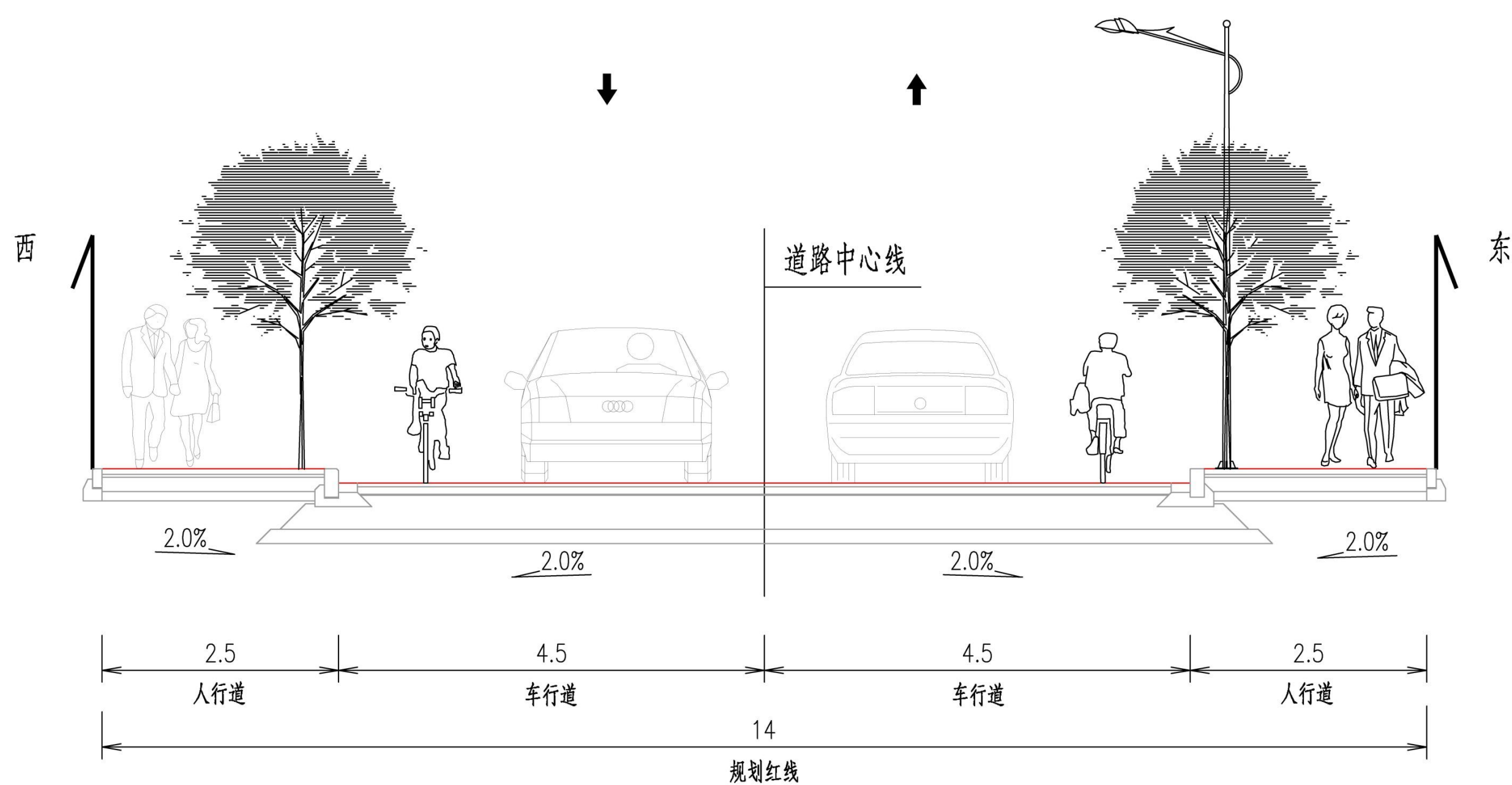
绿松路（永登路—武威路）道路标准横断面设计图
