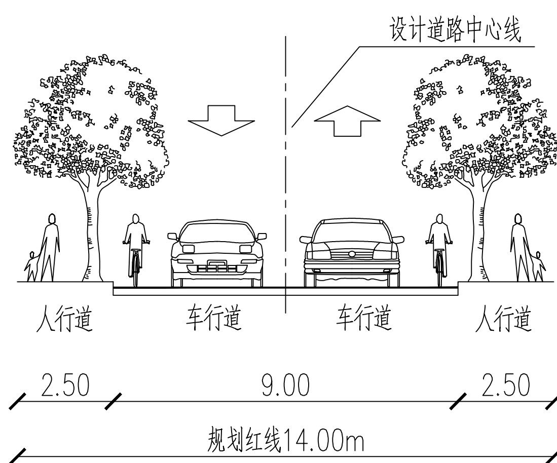
定宁路道路标准横断面 1:100
