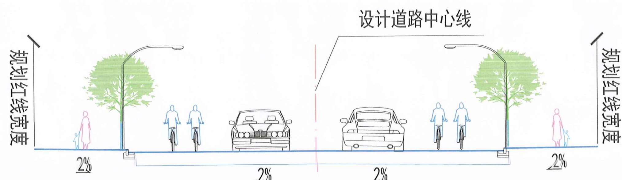
标准横断面设计图
